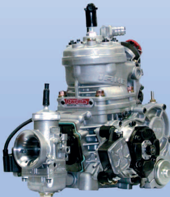
Reedster KF4 125
