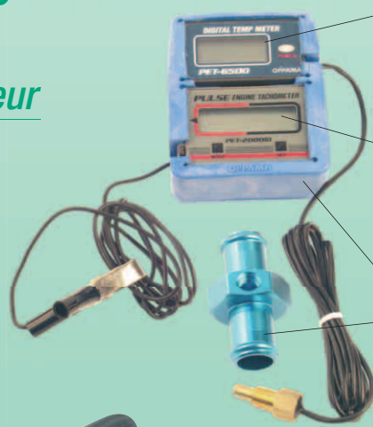
334150 = Water temp. indicator/ Temperaturmesser/ Indicateur de température PET 6500
